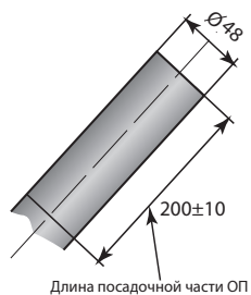
Рис. А.1 – Стандартное посадочное место консольных ОП
