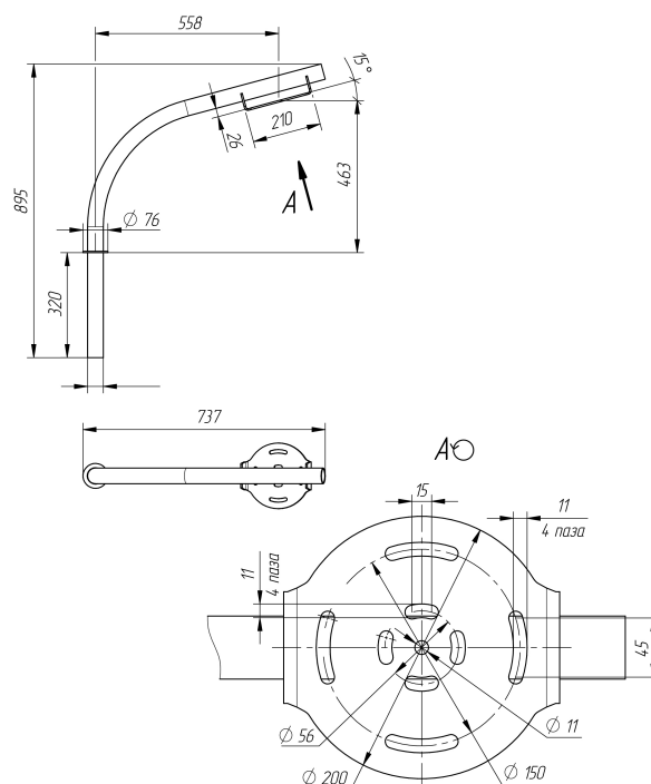
Кронштейн П1-0,5-0,5-Ф2-ц
