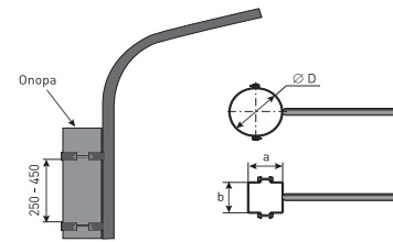
Рис. Б.3. — Характеристика установочных мест приставных кронштейнов (тип П)
