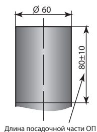
Рис. А.2 – Стандартное посадочное место торшерных ОП
