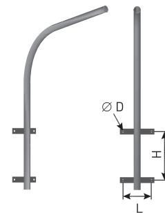
Рис. Б.4. — Характеристика установочных мест настенных кронштейнов (тип Н)
