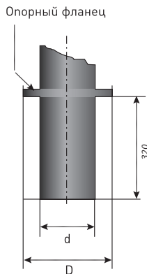
Рис. Б.2. — Характеристика установочных мест кронштейнов с фланцами (тип Ф)
