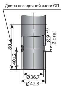
Рис. А.3 – Стандартное посадочное место подвесных ОП
