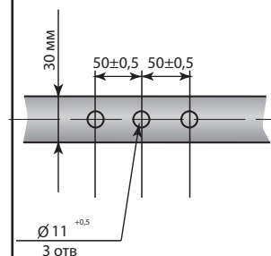
Рис. А.4 – Стандартное посадочное место прожекторов
