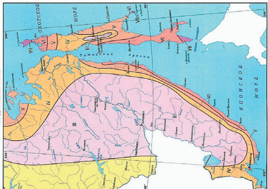
КАРТА 3а. РАЙОНИРОВАНИЕ ТЕРРИТОРИИ ПРИМОРСКОГО КРАЯ И ОСТРОВА САХАЛИН ПО ДАВЛЕНИЮ ВЕТРА
