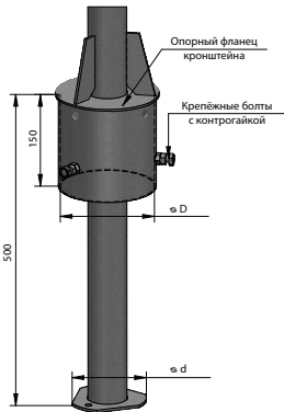
Рисунок Б.1. — Характеристика установочных мест кронштейнов с обечайками (тип О)
